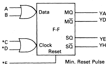
M291 — D Flip-Flop ½ Cell
